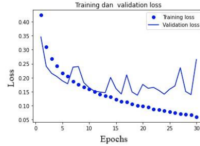
Gambar 32. Training Dan Validasi Loss Pada Suara On
