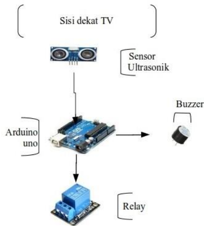
Gambar 2. Rancangan Perangkat Keras Dekat TV
