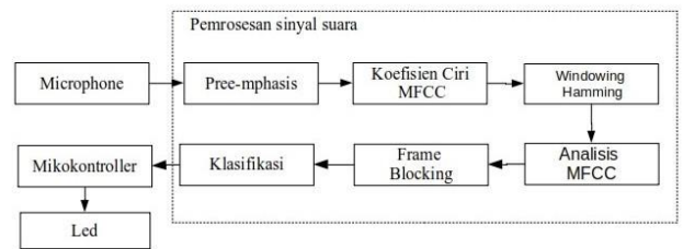
Gambar 5. Diagram Perancangan Sistem TV (Led) Dengan Inputan Suara
