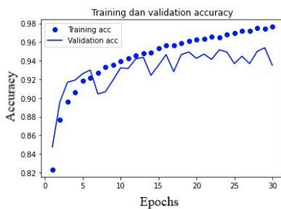
Gambar 11. Training Dan Validasi Akurasi Pada Suara On
